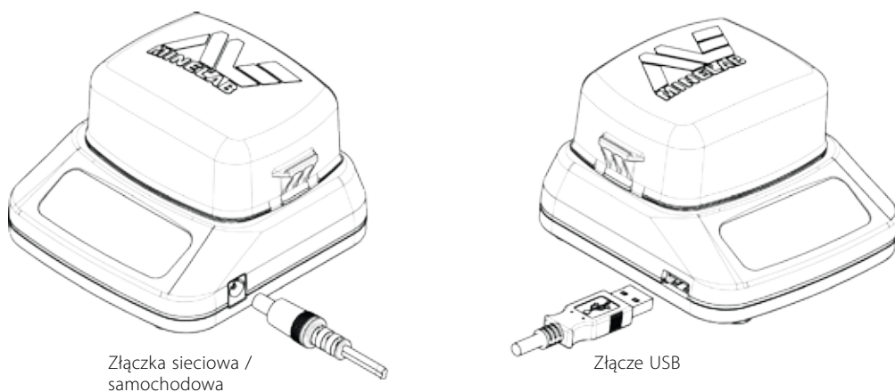
Ilustracja 36 – Ładowarka BC 10 z gniazdem na wtyczkę oraz złączem USB.
